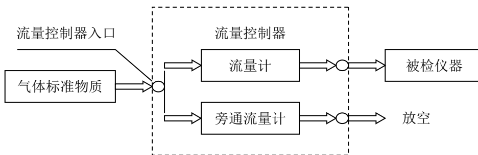
图 1 流量控制器示意图
