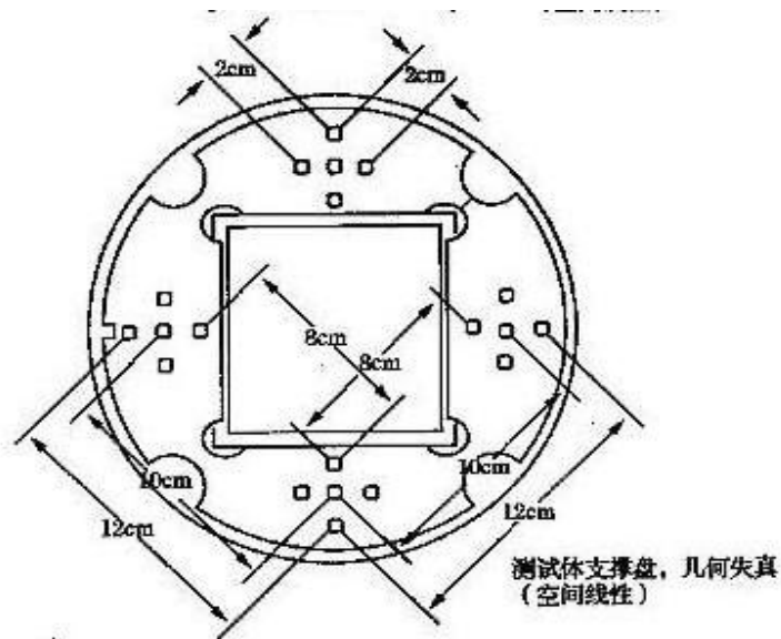
图 4 空间线性层
