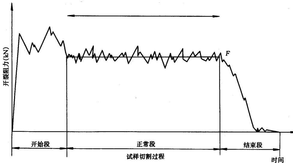
图 B3 开裂阻力的求取
