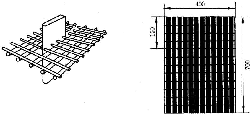
图 B1 试样切割示意图
