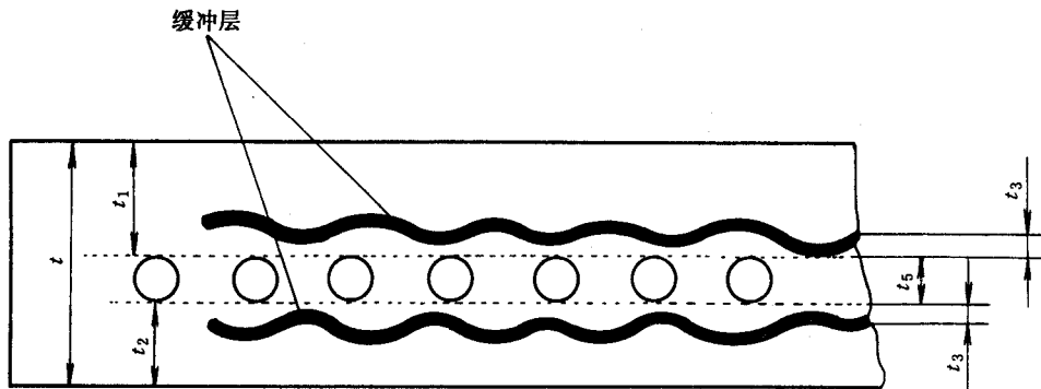
图 1 防撕裂带结构与尺寸
