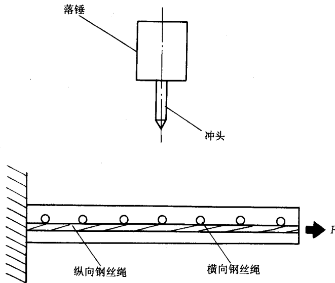
图 A1 试验装置示意图
