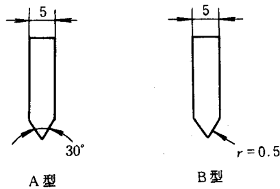
图 B2 刀具
