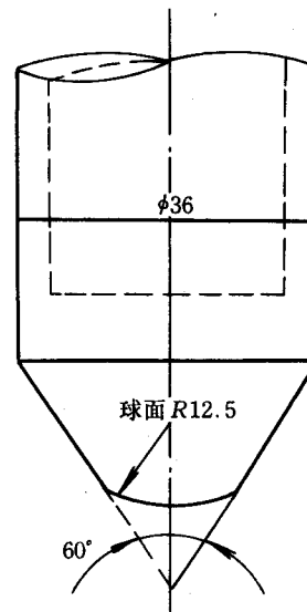
图 A2 冲头
