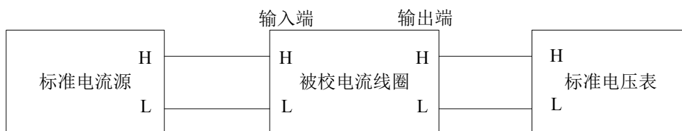
图 1 标准源法示意图
