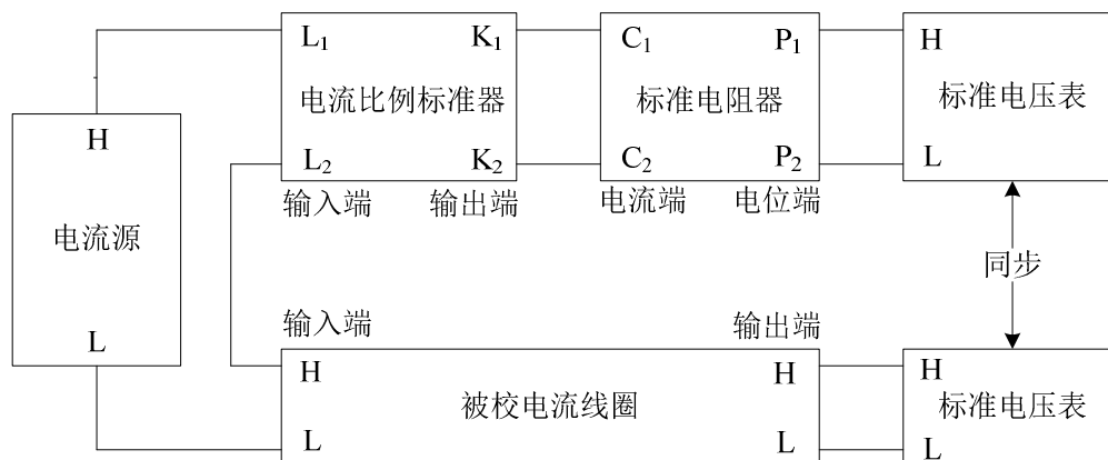
图2 标准表法示意图
